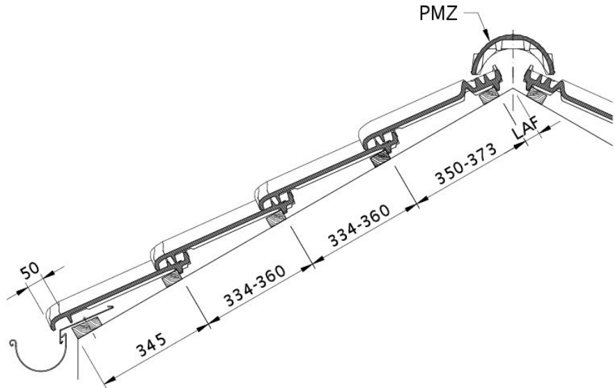
Technický výkres tašky MZ3 NEU DQF DQF
