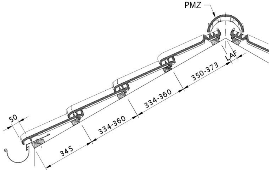
Technický výkres tašky MZ3 NEU DQF DQF
