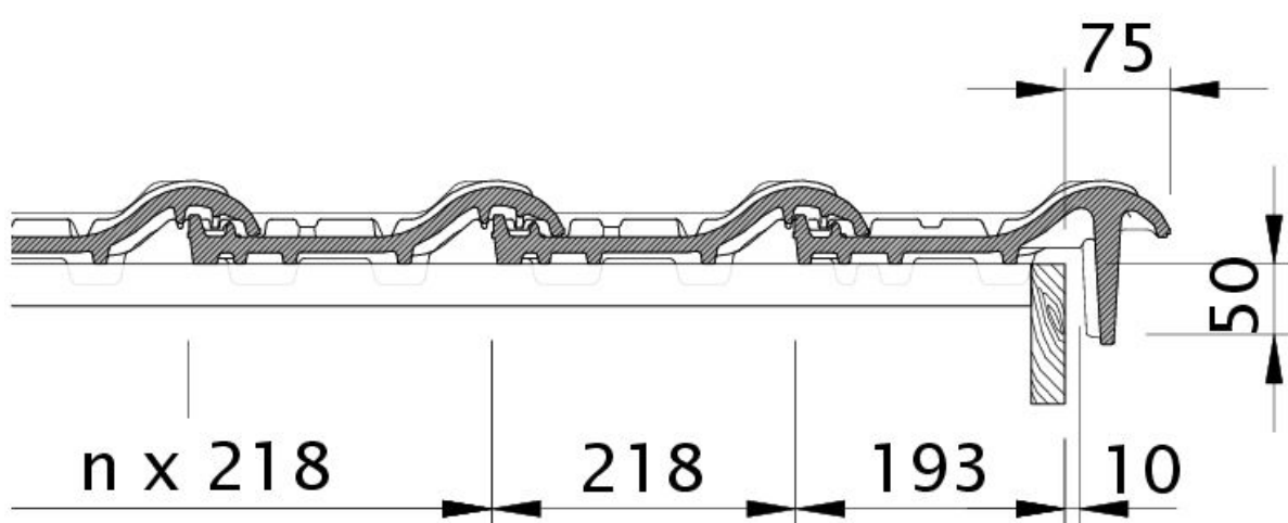
Technický výkres tašky MZ3 NEU OBL OBL
